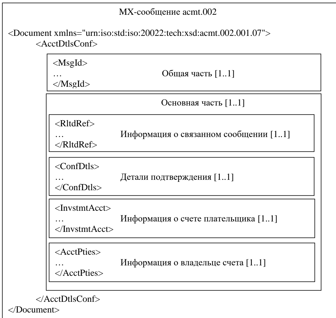
Рисунок 1 – Структура МХ-сообщения acmt.002
